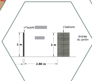
Coupe technique
