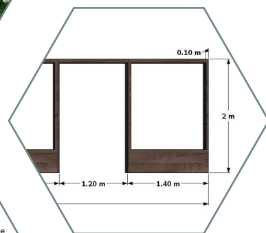
Détails techniques
